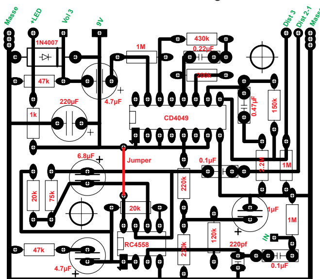
OD Dog Schéma de montage
